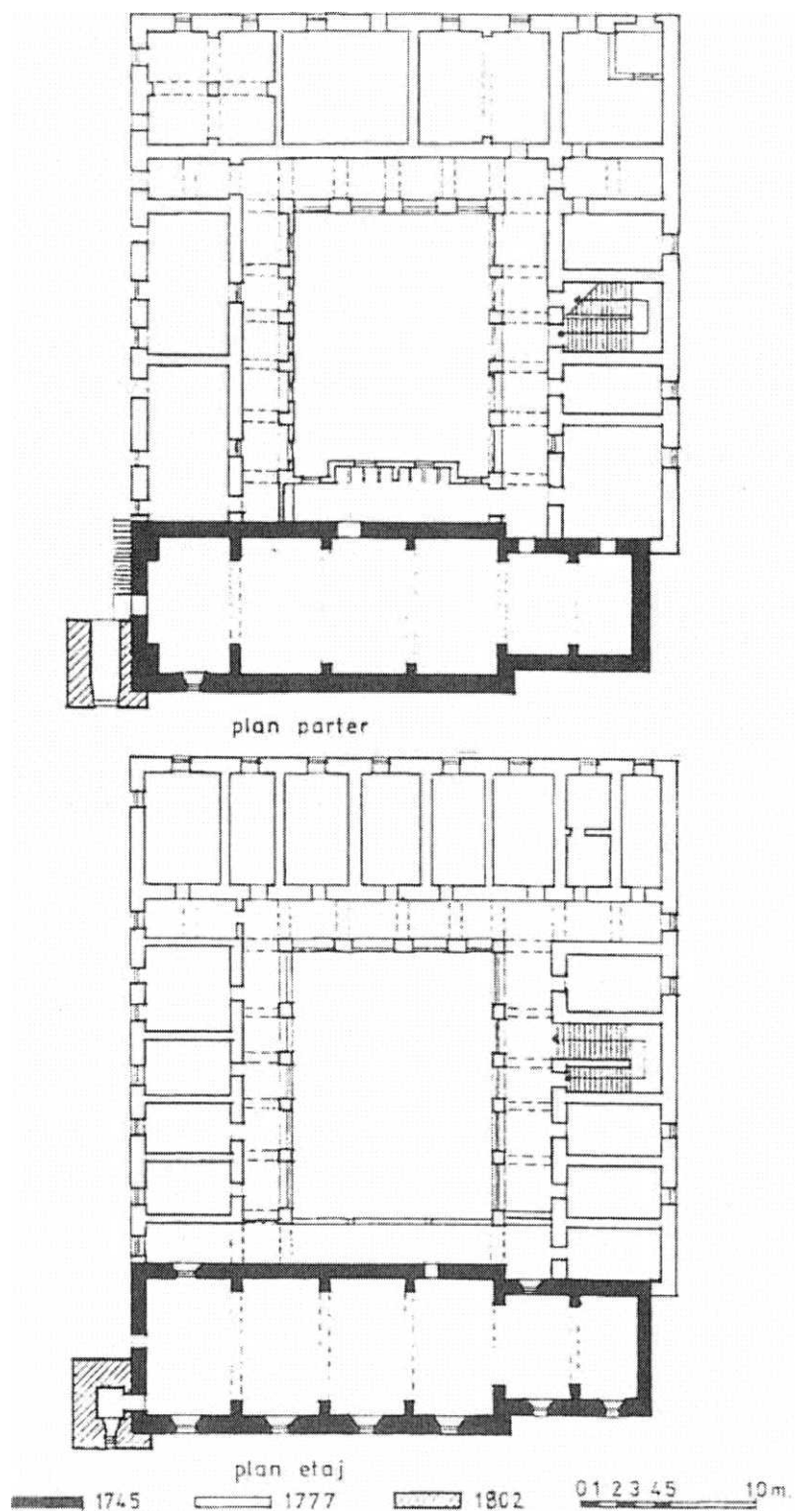
Fig. 83. Biserica cu mănăstirea franciscanilor, plan nivele.
