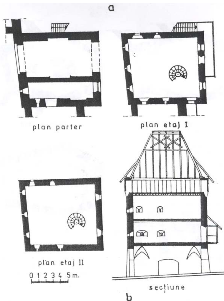
Fig. 35. Bastionul porții. a – Vedere generală; b – Planuri și secțiune.
