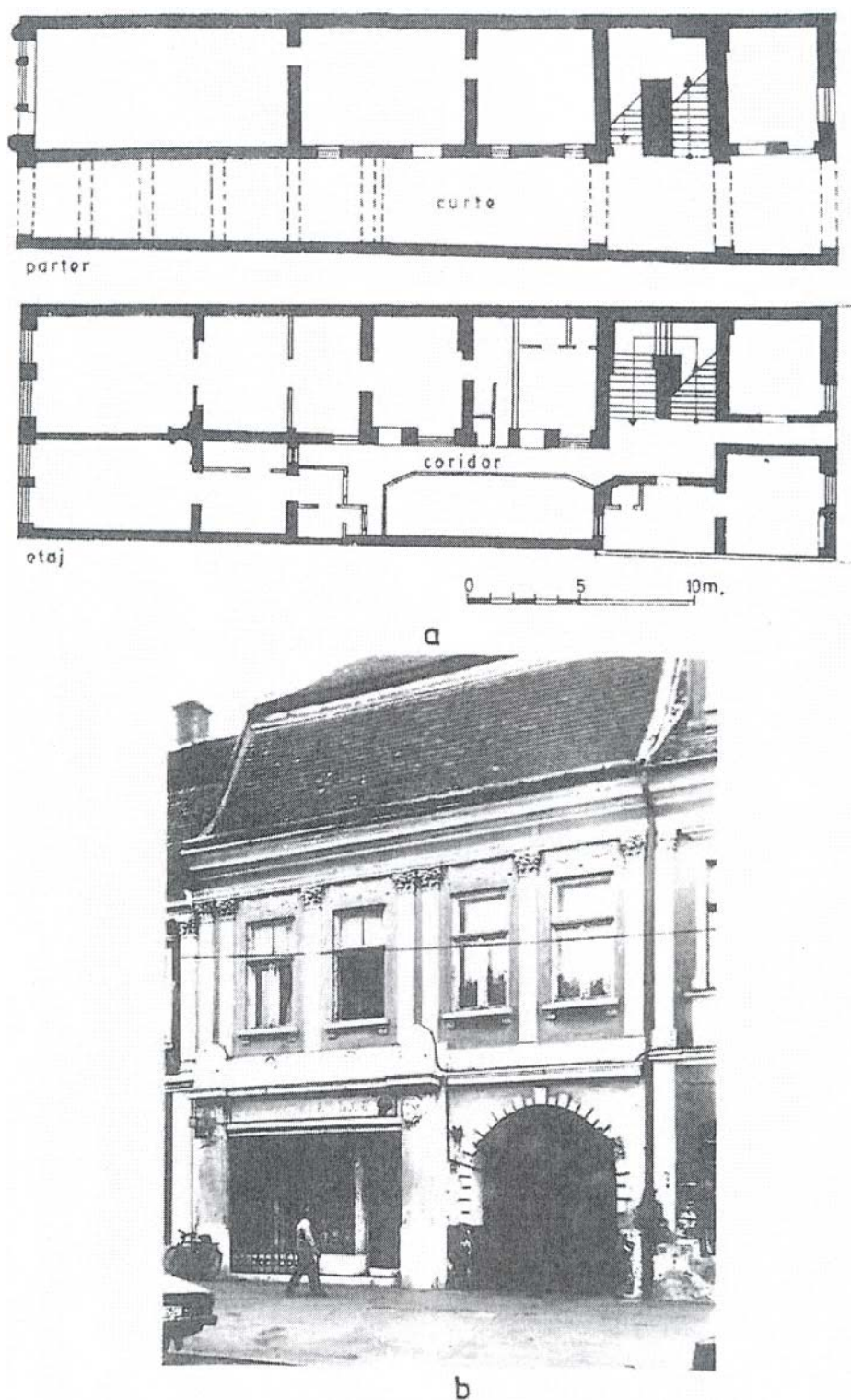
Fig. 112. Casa din Piața Trandafirilor nr. 55 (Casa Steibel). a – Plan nivele; b – Starea actuală.
