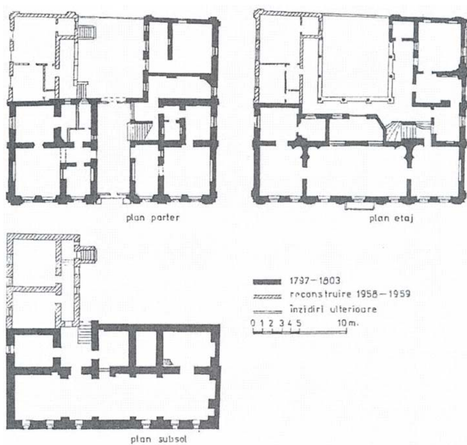
Fig. 105. Casa Teleki Domokos., plan nivele.
