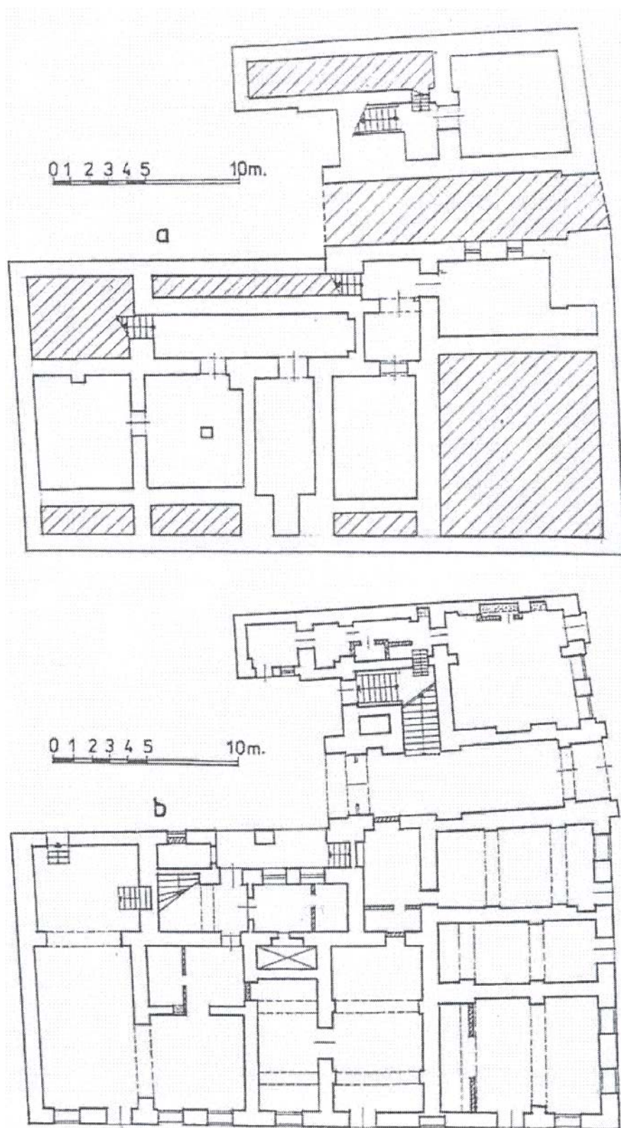
Fig. 51. Casa Köpeczi Tamás realizată în 1554. a – Plan subsol; b – Plan parter.
