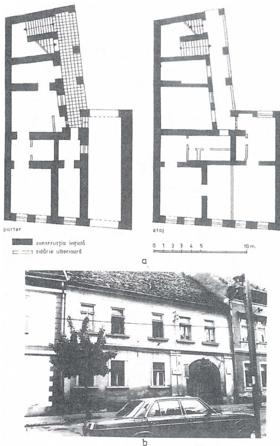
Fig. 113. Casa din str. Bolyai nr. 7. a – Plan nivele; b – Starea actuală.
