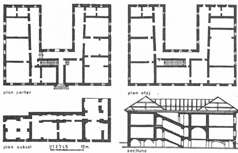
Fig. 79. Cazarma din cetatea orașului, plan nivele și secțiune
