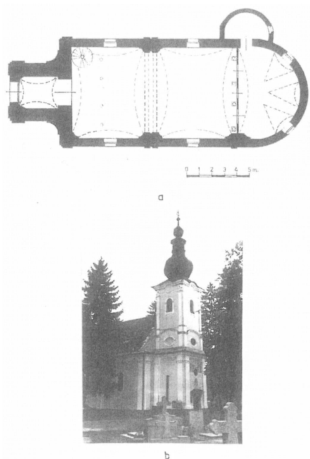
Fig.87. Biserica de piatră. a – Plan; b – Aspect general.
