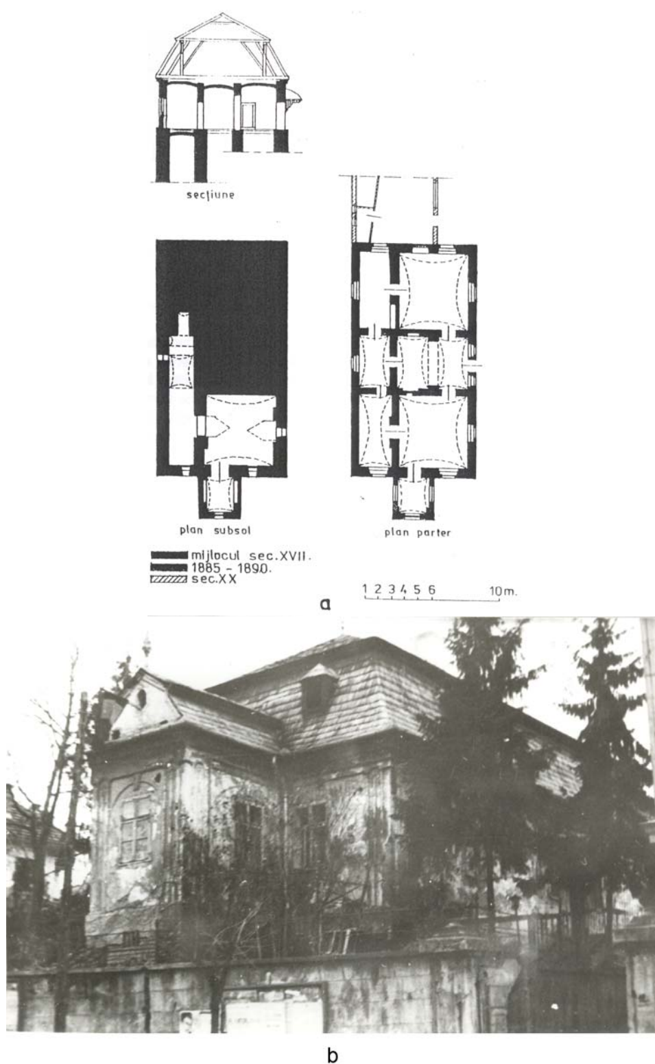
Fig. 54. Casa Pálffy. a – Plan nivele și secțiune; b – Aspect general.
