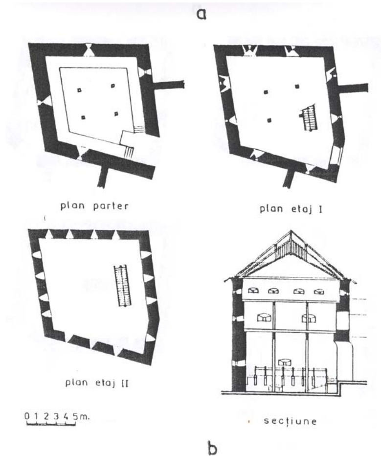
Fig. 39. Bastionul măcelarilor. a – Vedere generală; b – Planuri și secțiune.
