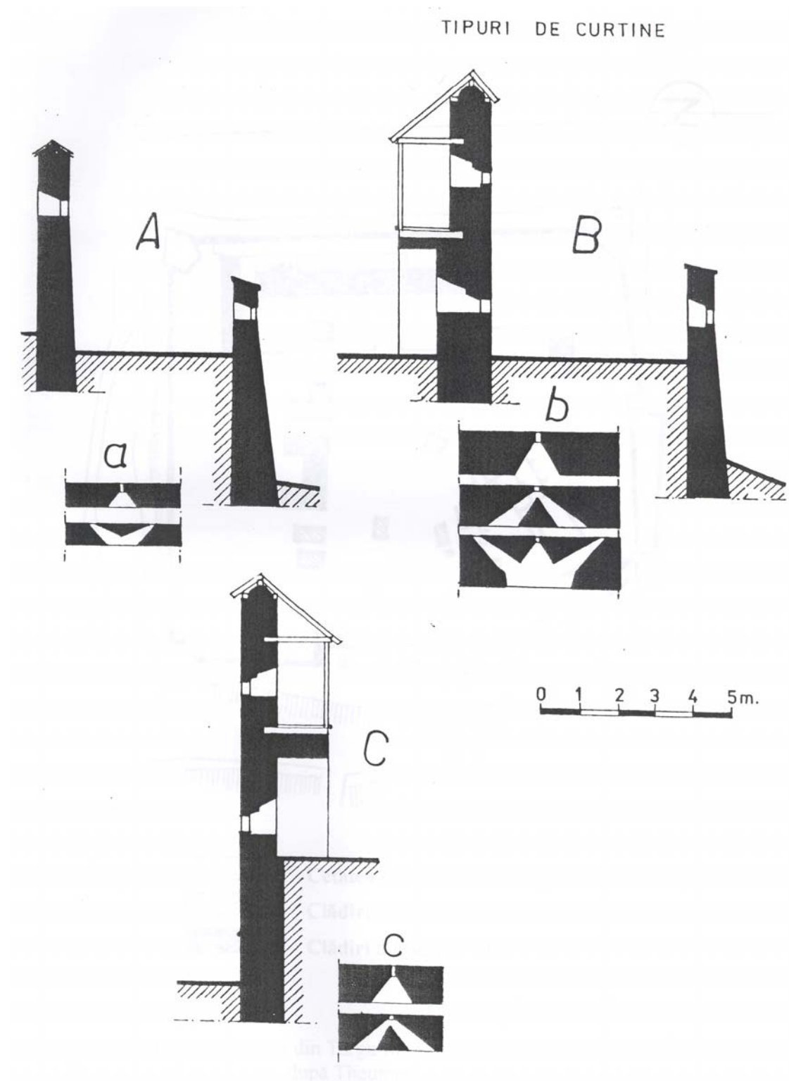
Fig. 41. Tipuri de cortine, secțiuni. A – Zwingerul situat între Bastionul tăbăcarilor și Bastionul mic; B – Curtina dublă dintre Bastionul mic și Bastionul porții; C – Curtina simplă din sistemul de apărare.
