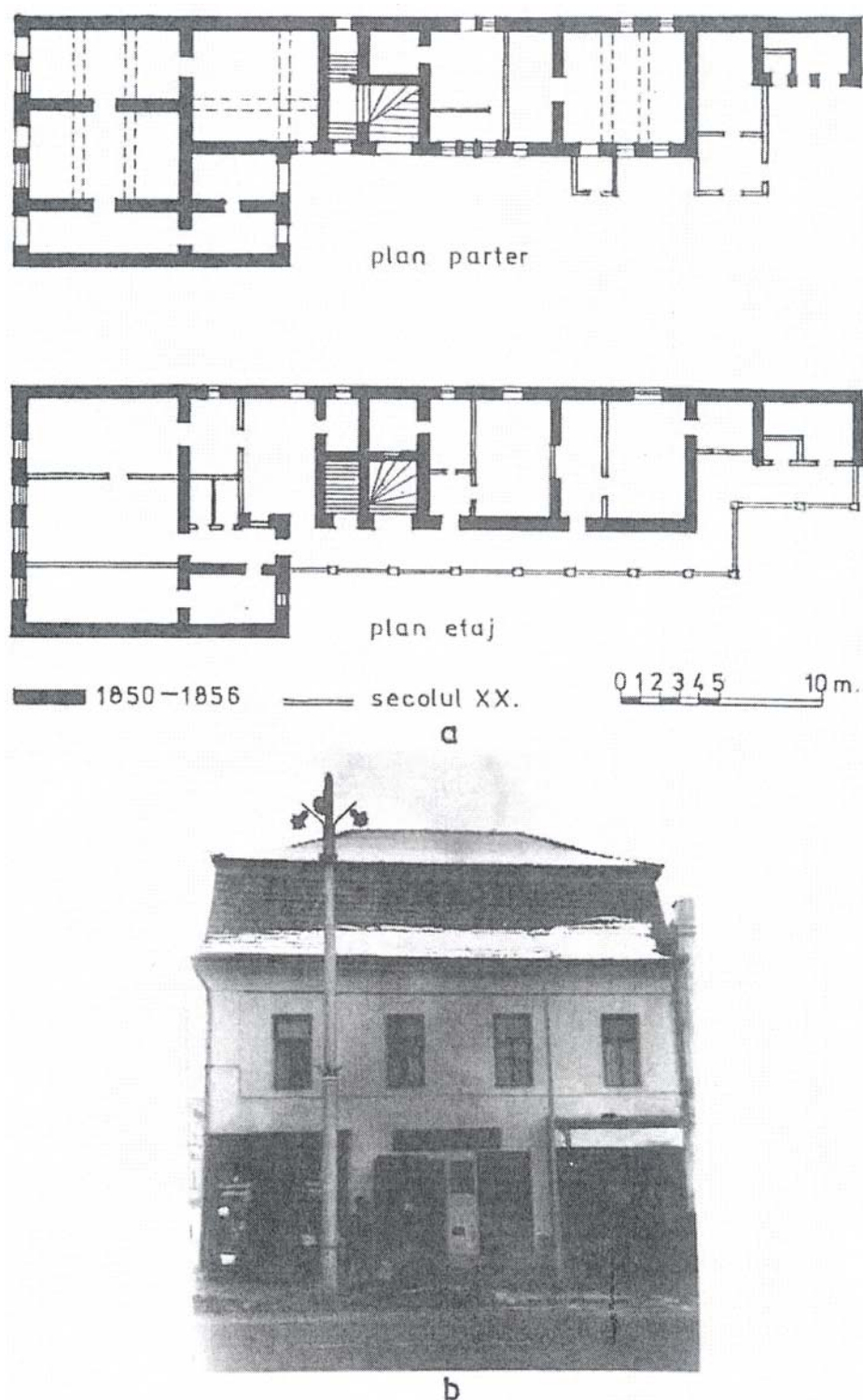
Fig. 115. Casa din Piața Trandafirilor nr. 58. a – Plan nivele; b – fațada principală înainte de modificările din anul 1973.
