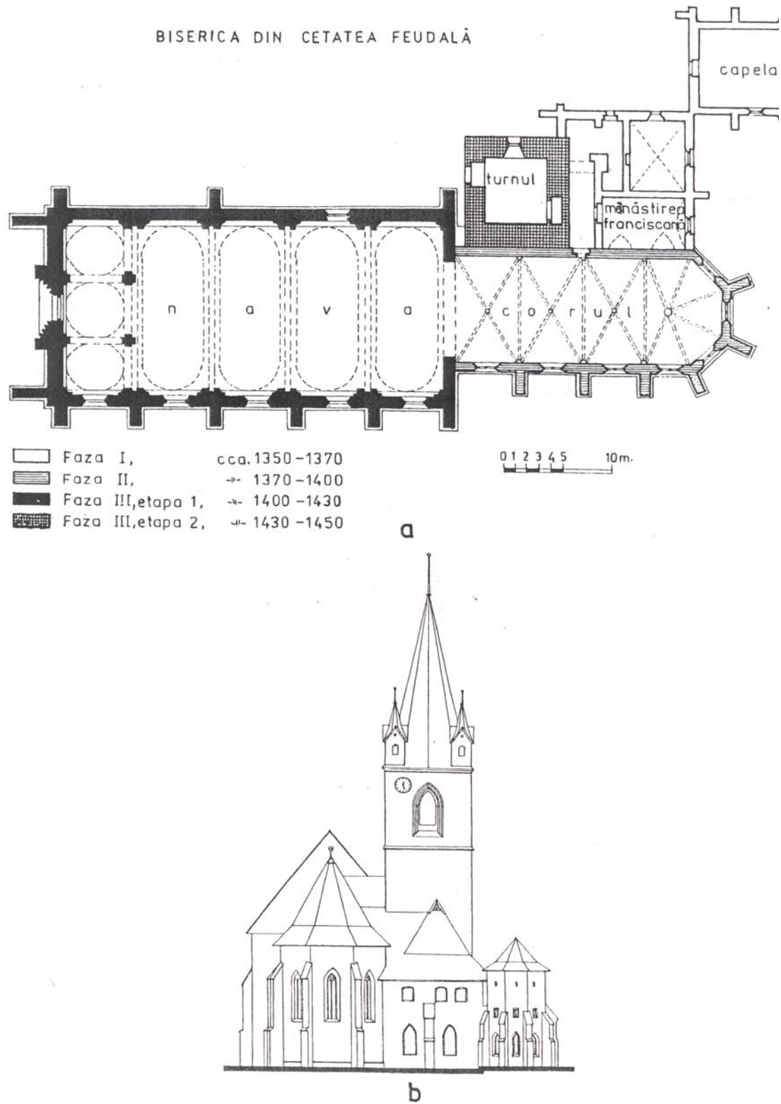
Fig. 43. Biserica gotică din cetate. a – Etapele constructive, plan; b – Capătul de vest al bisericii, desen.
