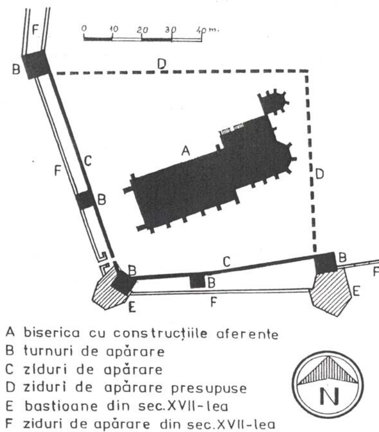
Fig. 30. Târgu-Mureș. Fortificația veche, plan.
