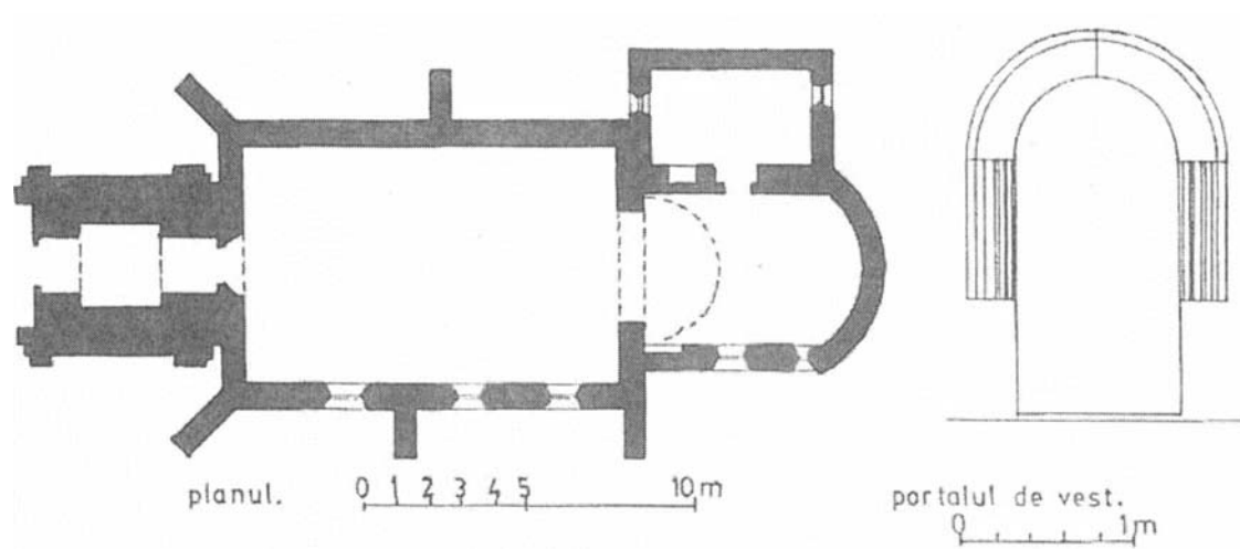
Fig. 29. Biserica romano-catolică din Sângeorgiu de Mureș, plan și detaliu.
