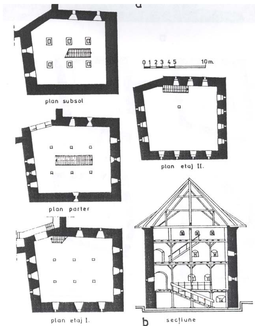
Fig. 38. Bastionul dogarilor. a – Vedere generală; b – Planuri și secțiune.
