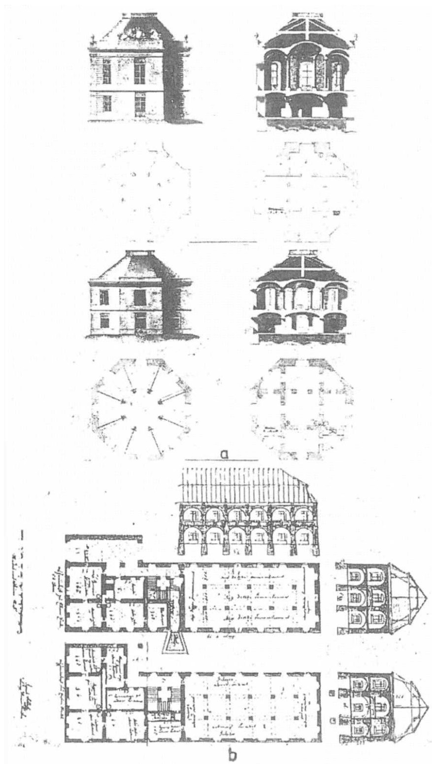
Fig. 97. Biblioteca Teleki. a – Proiectele lui Ugrai László. Plan nivele, fațade și secțiuni; b – Proiectul lui Schlaff Ignác, după care s-a realizat construcția. Plan nivele și secțiuni.
