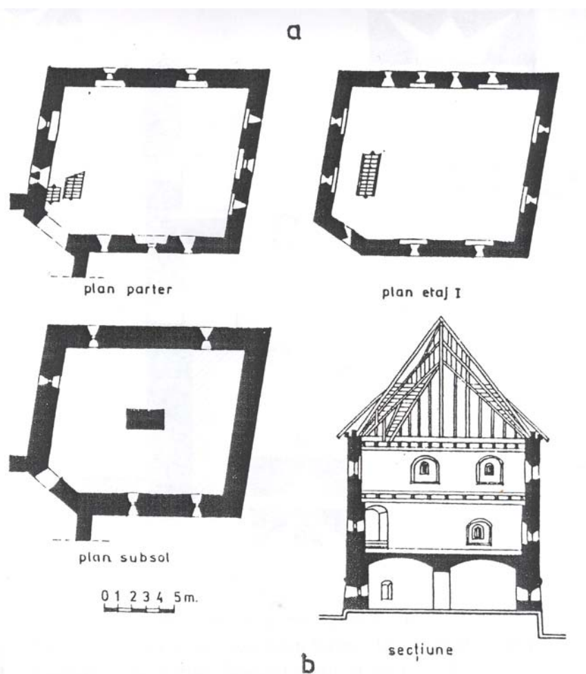
Fig. 40. Bastionul croitorilor. a – Vedere generală; b – Planuri și secțiune.
