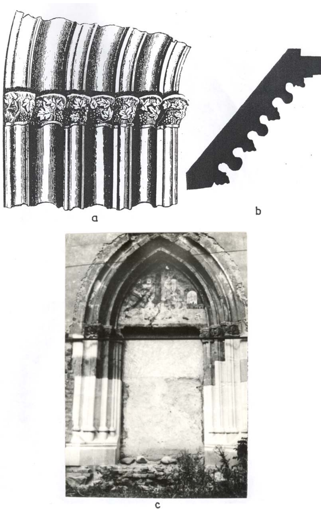
fig. 48. Biserica franciscană din cetate. a – Montanții portalului de vest, după Orbán Balázs; b – Secțiunea montanților, după Orbán Balázs; c- Portalul de sud, aspectul actual.
