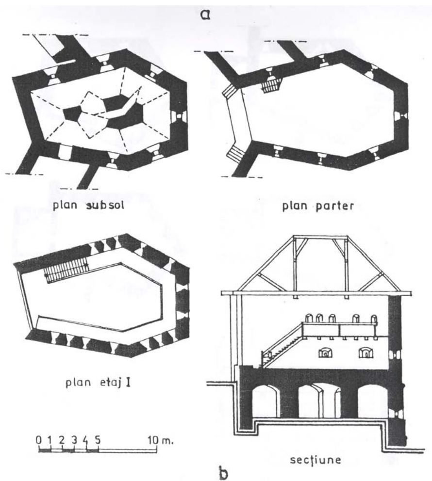
Fig. 36. Bastionul tăbăcarilor. a – Vedere generală; b – Planuri și secțiune.
