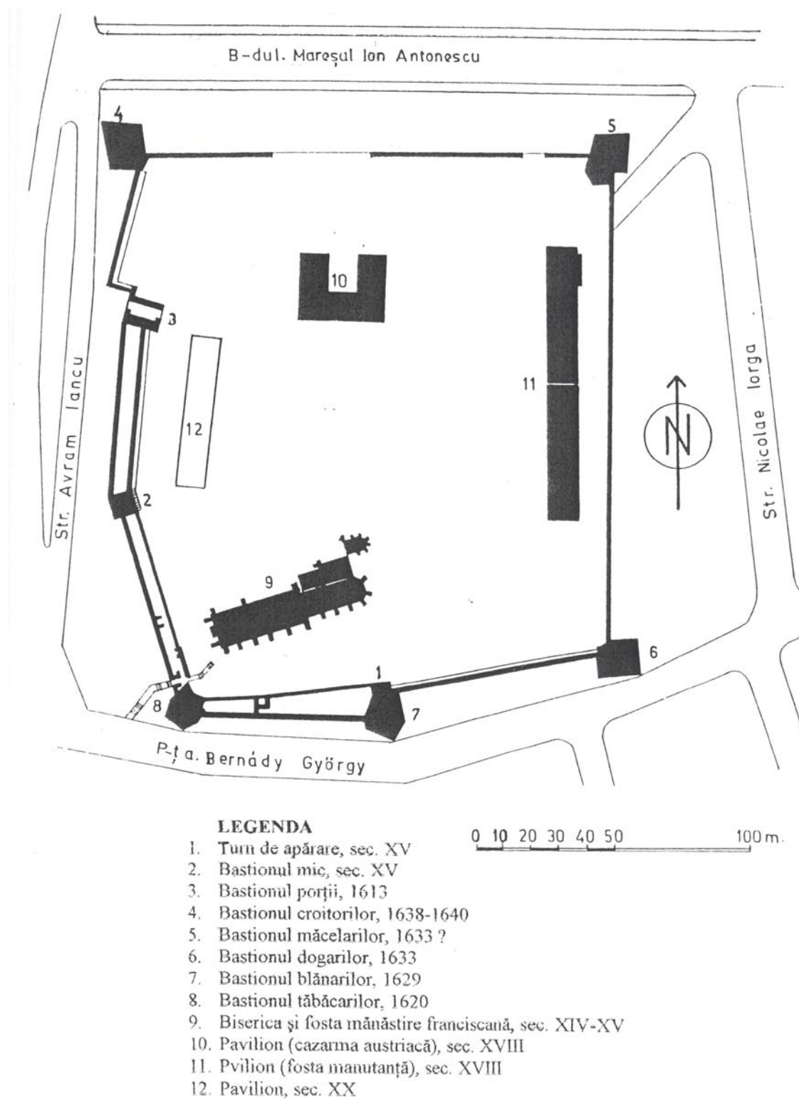
Fig. 34. Planul cetății secolului al XVII-lea.
