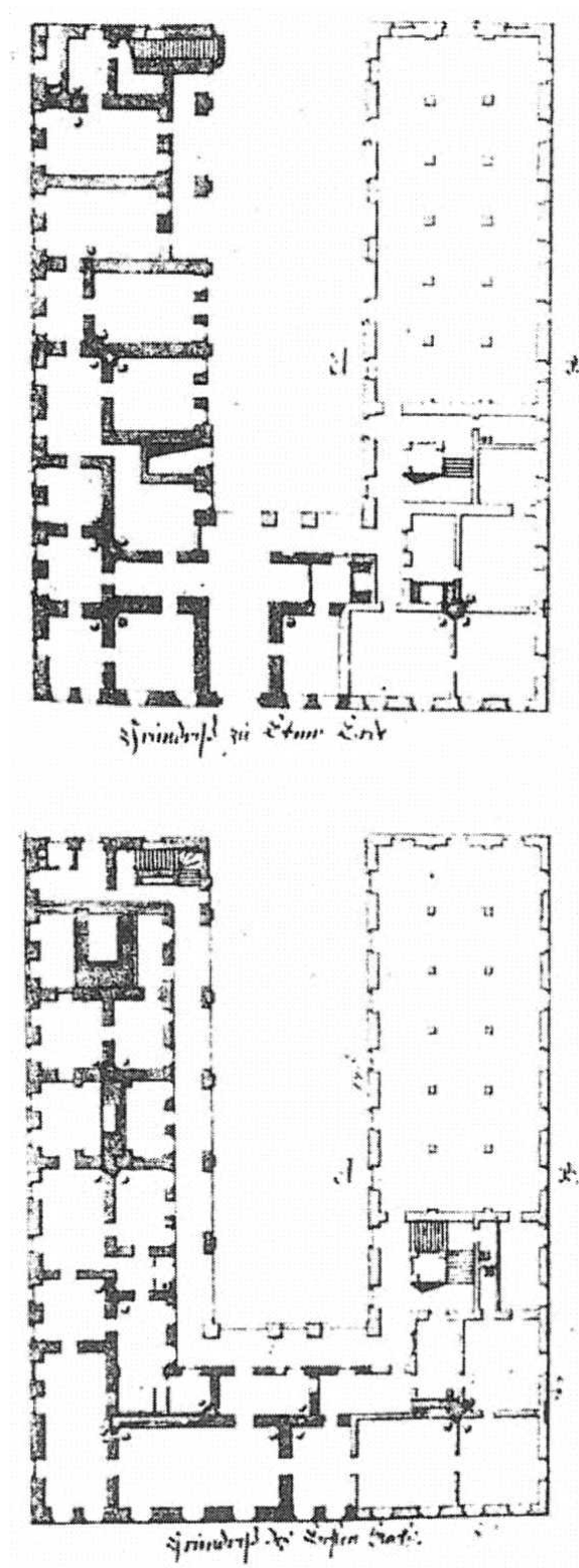
Fig. 96. Biblioteca Teleki. Proiectul lui Ernst Koch. Plan nivele.
