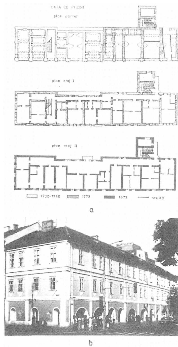
Fig. 88. Casa cu piloni. a – Plan nivele; b – Aspect general.
