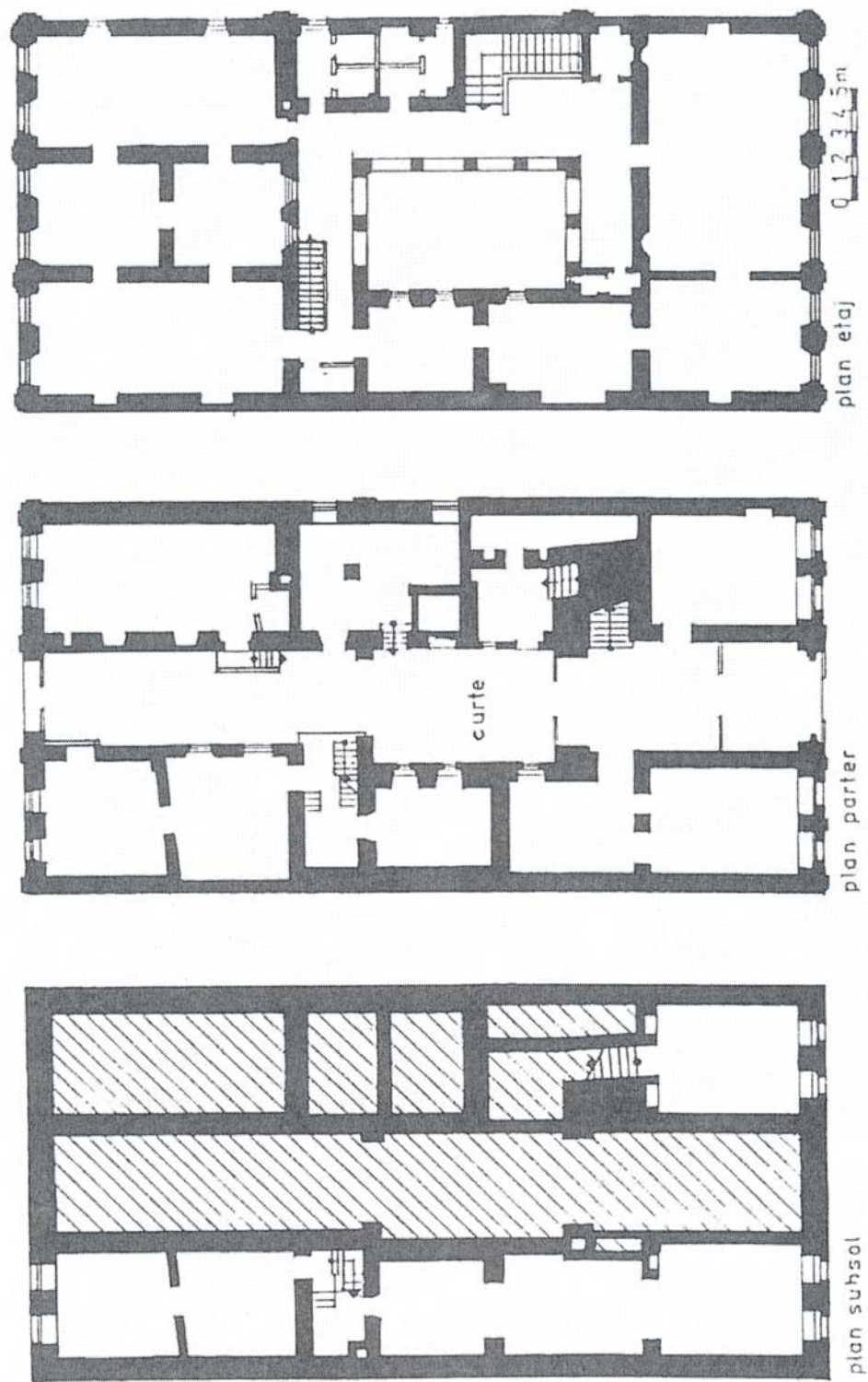
Fig. 101. Casa Toldalagi, plan nivele.
