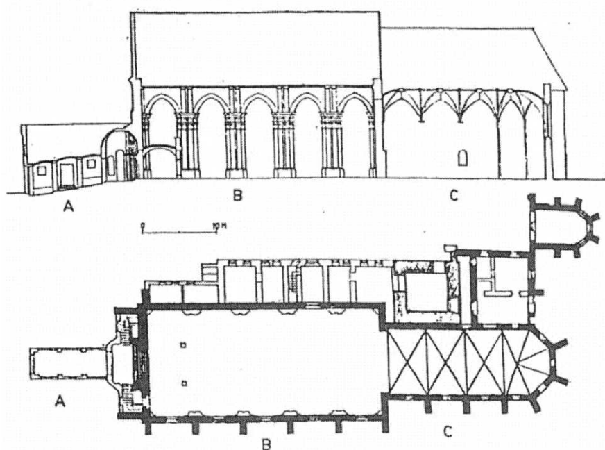
Fig. 80. Porticul dintre curtină și biserică, plan și secțiune. După Grigore Ionescu, în Istoria arhitecturii în România, I., București, 1963, p. 178, fig. 106. A – Porticul; B – Nava bisericii; C – Altarul-corul.
