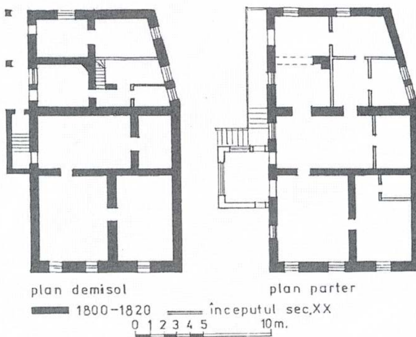
Fig. 116. Casa din strada Avram Iancu nr. 23. a – Aspect actual; b – Plan nivele.
