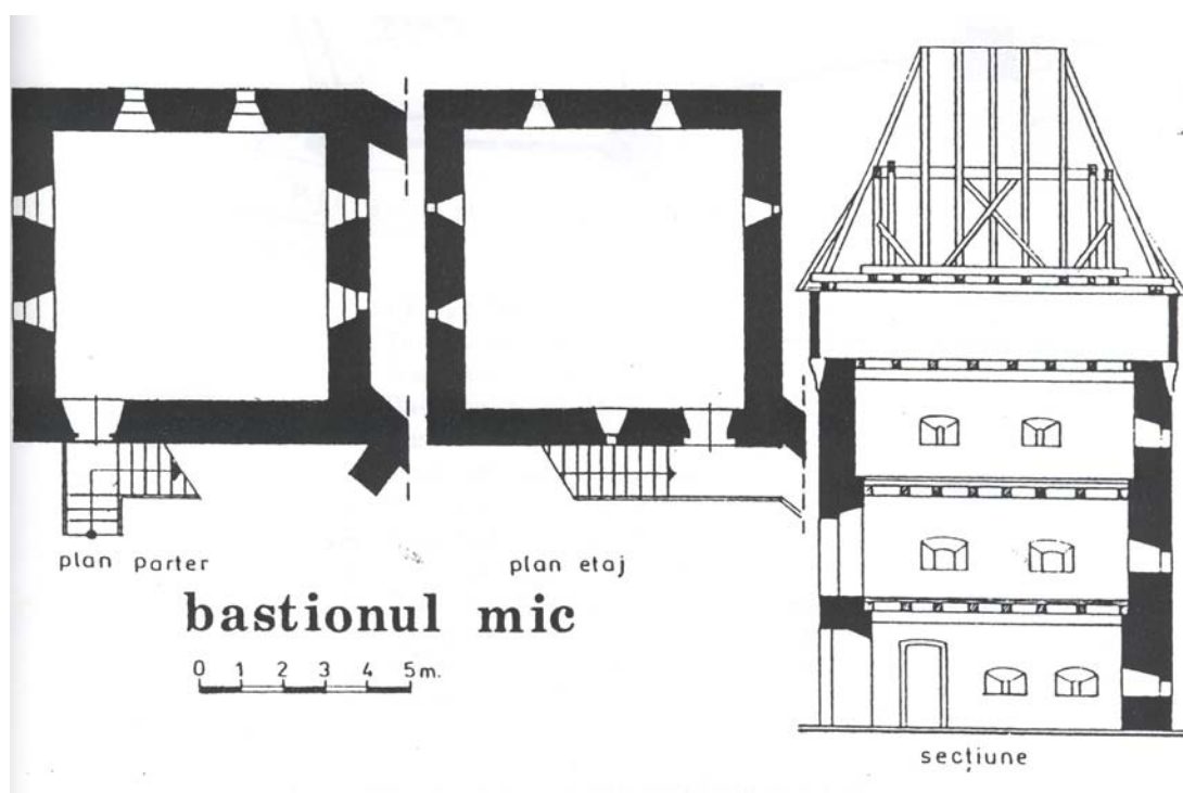
Fif. 33. Turnul mic, plan nivele și secțiune.
