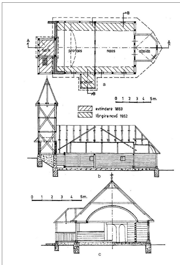
Biserica de lemn de la Romăneni, cu hramul „Intrarea în biserică a Maicii Domnului” Proiectul de renovare din anul 1975. a – Plan; b – Secțiune longitudinală; c- Secțiune transversală 10
