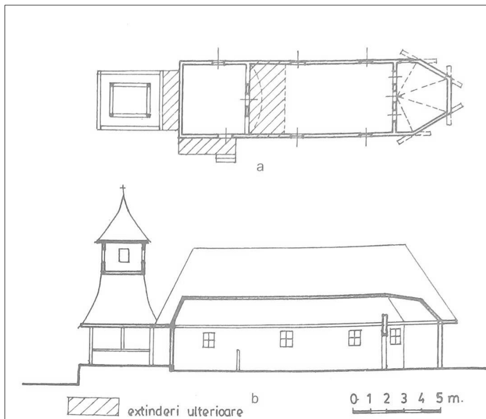
Biserica de lemn de la Româneeni, cu hramul „Intrarea în biserică a Maicii Domnului”, a – Plan; b – Secțiune longitudinală 9
