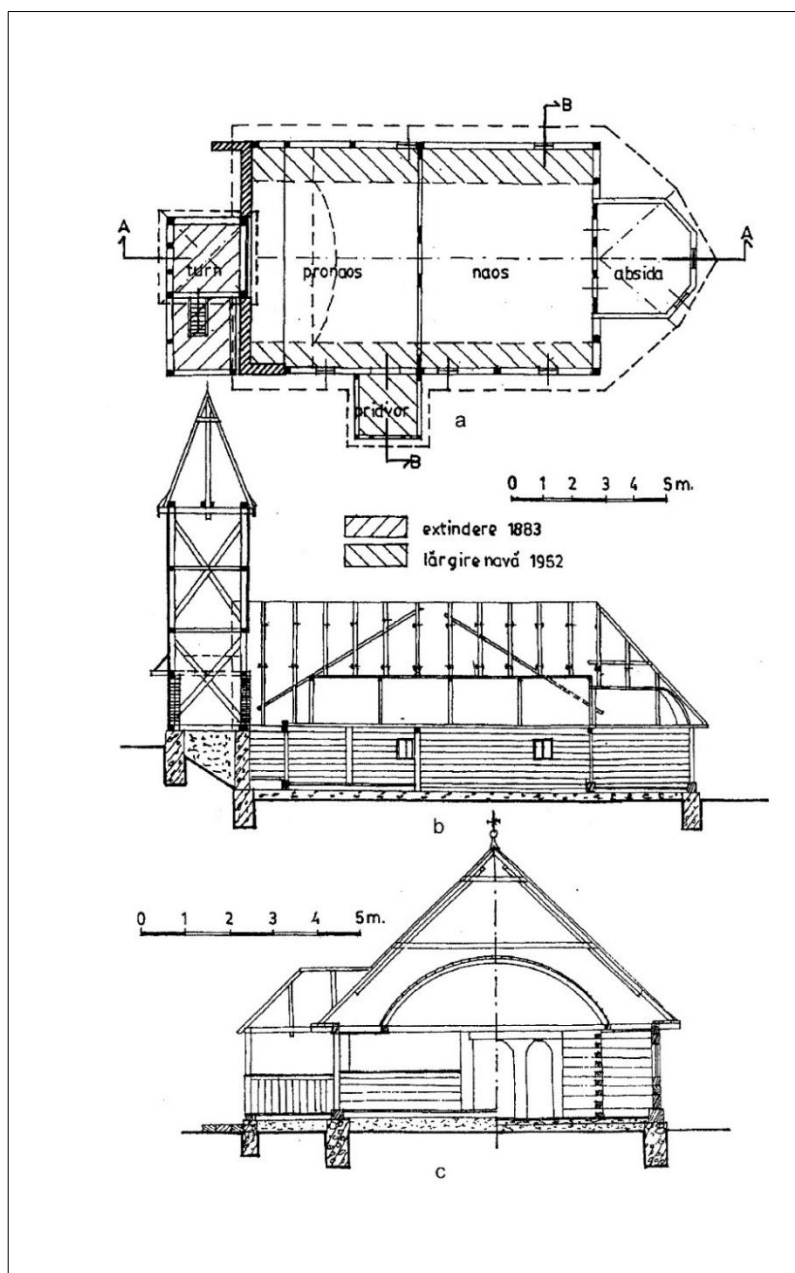
Oroiu. Biserica „Sfinții Arhangheli”, după proiectul de renovare. a – Plan; b – Secțiune longitudinală; c – Secțiune transversală
